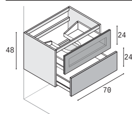
Waschtisch-Unterschrank mit 1 Obere-Auszug mit schwarzem Aluminiumrahmen + Stop-sol-Glas, 1 Untere-Auszug.
