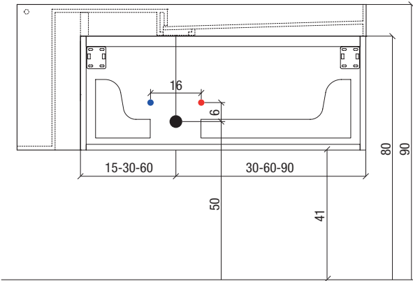
Waschtisch WRAP 1, Becken mit 1 Armaturenbohrung an der Seite (Beispiel)
