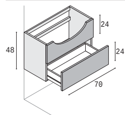
Waschtisch-Unterschrank für Halbeinbau-Waschtische mit 1 festen Frontblende, 1 Auszug.
