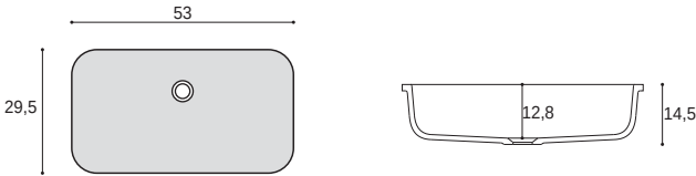
RETTANGOLARE 53 x 29,5 cm für Waschtisch-Unterschranke ≥ 70
