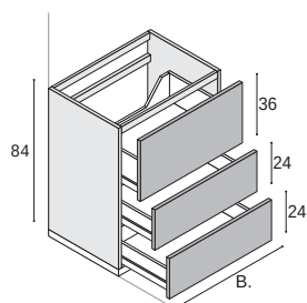
Waschtisch-Unterschrank mit 3 Auszügen.
