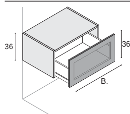
Unterschrank mit 1 Auszug mit schwarzem Aluminiumrahmen + Stop-sol-Glas.
