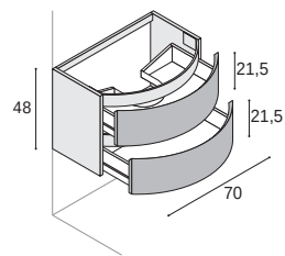
Waschtisch-Unterschrank mit 2 Auszügen gerundet.
