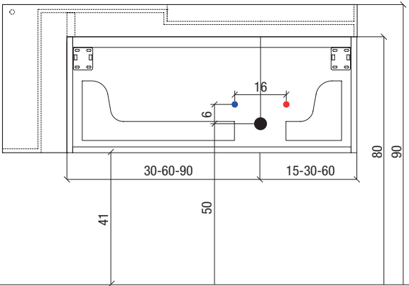
Waschtisch WRAP 2, Becken mit 1 Armaturenbohrung hinten mittig (Beispiel)
