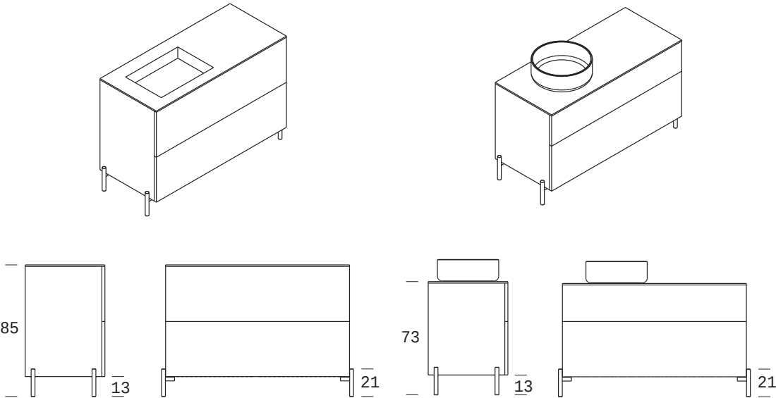
H.72 FUGENLOSE WASCHTISCHE
