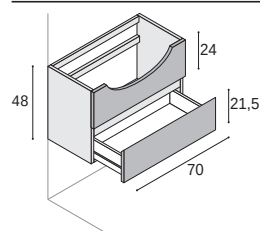
Waschtisch-Unterschrank für Halbeinbau-Waschtische mit 1 festen Frontblende, 1 Auszug.
