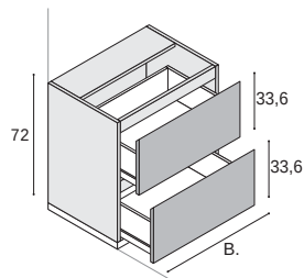
Unterschränk mit 2 Auszügen.
