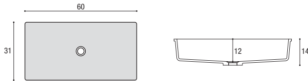
RETTANGOLARE 60 x 31 cm für Waschtisch-Unterschranke ≥ 70
