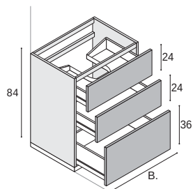
Waschtisch-Unterschrank mit 3 Auszügen.
