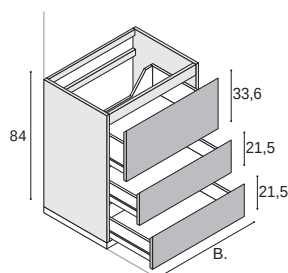
Waschtisch-Unterschrank mit 3 Auszügen.
