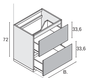
Waschtisch-Unterschrank mit 2 Auszügen. Empfohlen für Auflegewaschtische.
