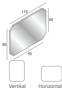
Spiegel OTTAGONO BIG. Ohne Schalter / Steckdose.
