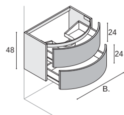
Waschtisch-Unterschrank mit 2 Auszügen gerundet.
