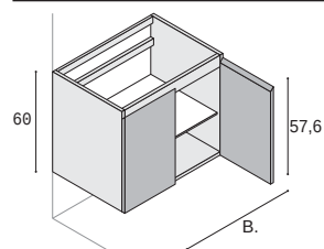
Waschtisch-Unterschrank mit 2 Türen, 1 Glas-Einlegeboden (fix, durchgehend).
