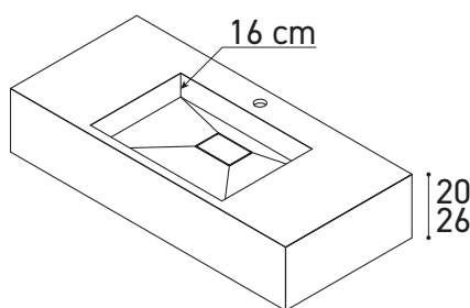
Beispiele für asymmetrische Beckenplatzierungen der Becken META, auch bis direkt an den Waschtischrand.
