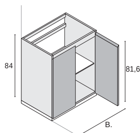
Waschtisch-Unterschrank mit 2 Türen, 1 Glas-Einlegeboden (fix, durchgehend).
