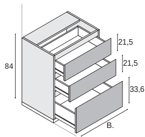
Unterschrank mit 3 Auszügen.
