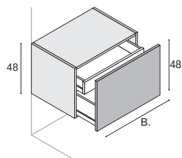
Unterschrank mit 1 Auszug + 1 Schublade innen.
