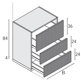
Unterschrank mit 3 Auszügen.
