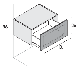
Unterschrank mit 1 Auszug mit schwarzem Aluminiumrahmen + Stop-sol-Glas.
