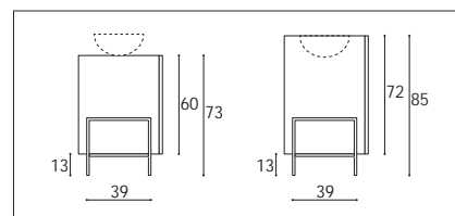
STRUCTURA-Element Höhe 35 cm (beidseitig verwendbar) mit Unterschrank H 60 (mit Auflagebecken) bzw. H 72 cm (mit fugenlosem Waschtisch)
