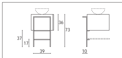
STRUCTURA-Element Höhe 68 cm (beidseitig verwendbar) mit Unterschrank H 36 cm mit Auflagebecken
