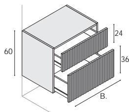
Unterschrank mit 2 Auszügen.
