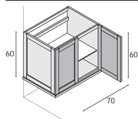
Waschtisch-Unterschrank mit 2 Türen, 1 Glas-Einlegeboden (fix, durchgehend).
