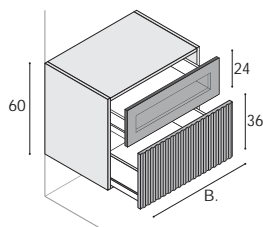
Unterschrank mit 1 Obere-Auszug mit schwarzem Aluminiumrahmen + Stop-sol-Glas, 1 Untere-Auszug. Glasfront nur mit PROFILO-Griff Schwarz kompatibel. KEIN Push-Pull.
