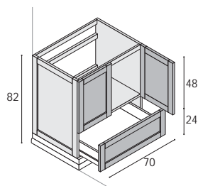
Waschtisch-Unterschrank mit 2 Türen, 1 Glas-Einlegeboden (fix, durchgehend).
