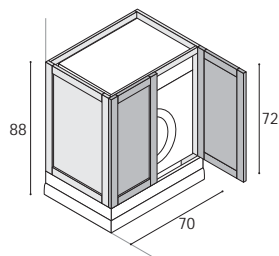
Waschmaschinen-Unterschrank mit 2 Türen.
