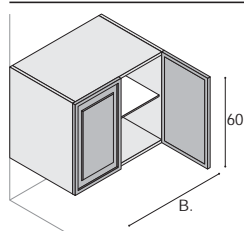
Unterschränk mit 2Türen, 1 Glas-Einlegeboden (fix, durchgehend).
