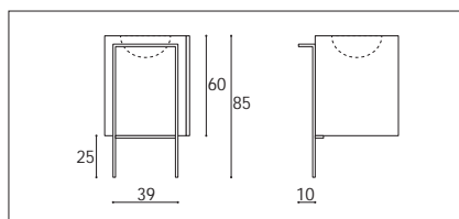
STRUCTURA-Element Höhe 80 cm (beidseitig verwendbar) mit Unterschrank H 60 cm mit fugenlosem Waschtisch
