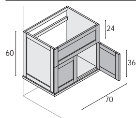
Waschtisch-Unterschrank mit einer Frontblende fix, 2 Türen,
