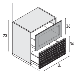
Unterschränk mit 1 Obere-Auszug mit schwarzem Aluminiumrahmen + Stop-sol-Glas, 1 Untere-Auszug. Glasfront nur mit PROFILO-Griff Schwarz kompatibel. KEIN Push-Pull.
