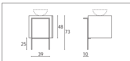
STRUCTURA-Element Höhe 68 cm (beidseitig verwendbar) mit Unterschrank H 48 cm mit Auflagebecken
