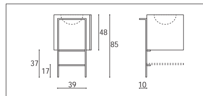
STRUCTURA-Element Höhe 80 cm (beidseitig verwendbar) mit Unterschrank H 48 cm mit fugenlosem Waschtisch
