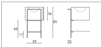
STRUCTURA-Element Höhe 80 cm (beidseitig verwendbar) mit Unterschrank H 36 cm mit fugenlosem Waschtisch
