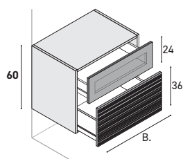
Unterschränk mit 1 Obere-Auszug mit schwarzem Aluminiumrahmen + Stop-sol-Glas, 1 Untere-Auszug. Glasfront nur mit PROFILO-Griff Schwarz kompatibel. KEIN Push-Pull.
