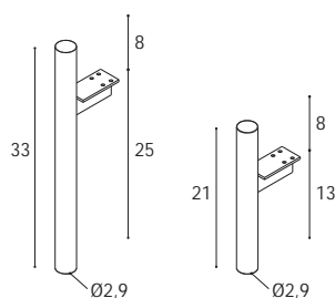
VERTIGO Einstellfuß, aus röhrenförmigem Metall mit Stützhalterung und Regulierungsmöglichkeit
