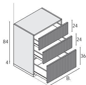
Unterschränk mit 3 Auszügen.
