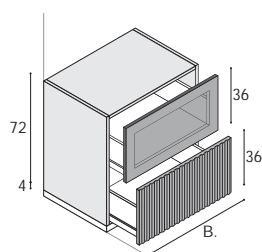
Unterschrank mit 1 Obere-Auszug mit schwarzem Aluminiumrahmen + Stop-sol-Glas, 1 Untere-Auszug. Glasfront nur mit PROFILO-Griff Schwarz kompatibel. KEIN Push-Pull.
